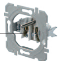
vijačna pritrditev vodnikov screw contacts
